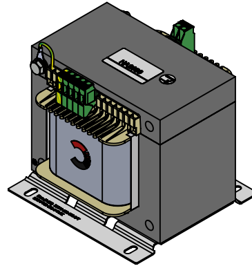
HA2090 PRI 380-400-420V SEC 230V 2000VA
