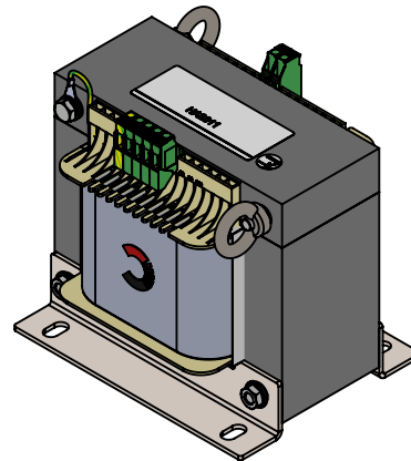
HA2911 PRI 380-400-420V SEC 230V 2500VA
